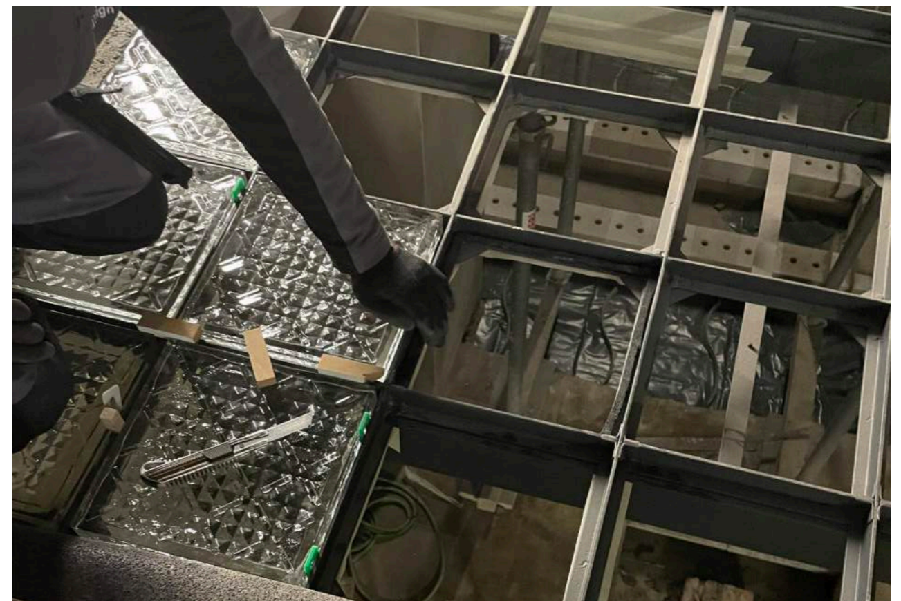
Betongläser Sonderanfertigung, 27,6 x 29,6 x 2,85 cm und 29,6 x 29,6 x 2,85 cm klassische Verlegung, FlexFuge-Verlegesystem Fußboden/Decke eines ehemaligen Tresors Mauerstraße, BMG Berlin, Deutschland 2022
