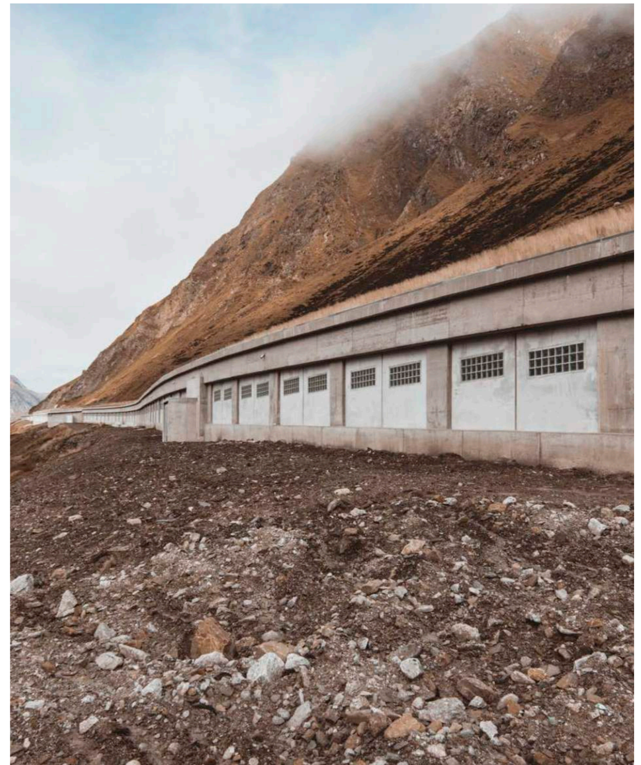
F30 Vollsicht, 19 x 19 x 10 cm, Montage von in unserem Werk hergestellten Fertigelementen Lawinenschutzwand Scopi, Schweiz Außenwand 2,6 km 2019
